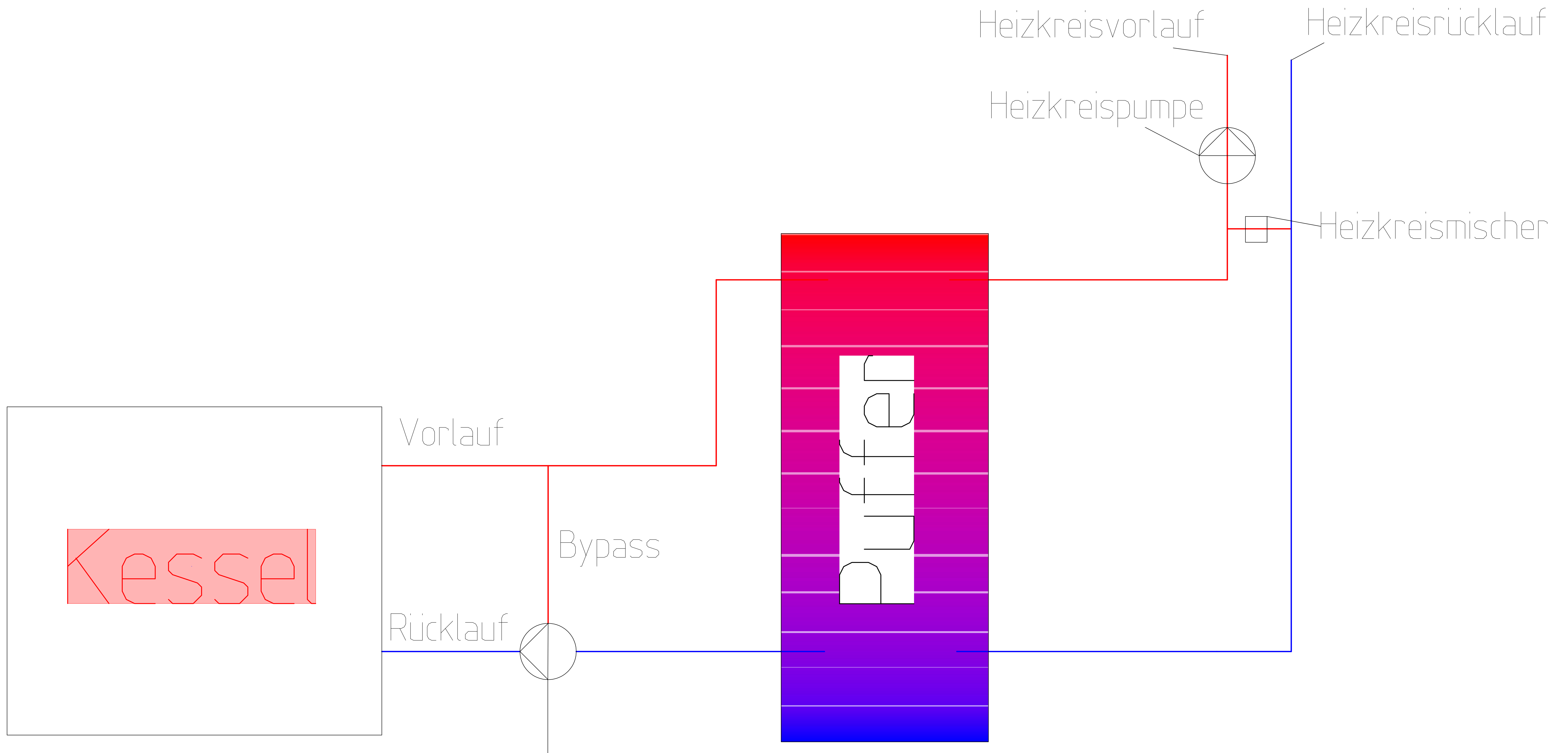
3-Wege-Ventil mit Ladepumpe
