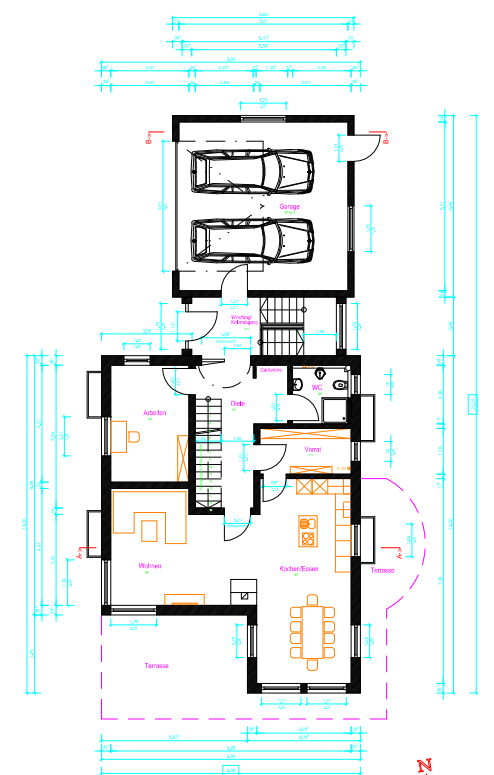
GRUNDRISS ERDGESCHOSS
