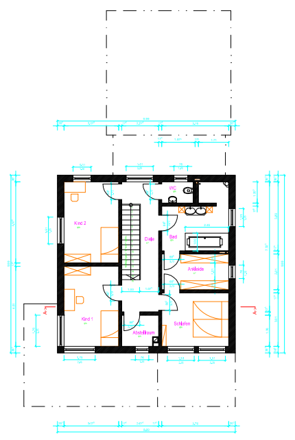
GRUNDRISS OBERGESCHOSS
