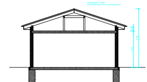
SCHNITT B-B
